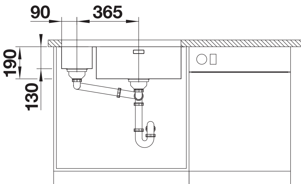
Vooraanzicht
