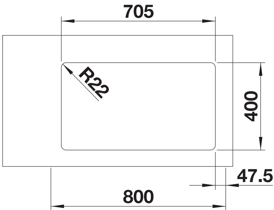
Uitsparing
