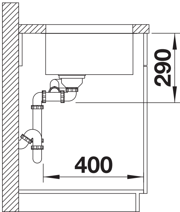
Zijaanzicht
